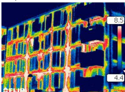
Mise en évidence des différents ponts thermiques
